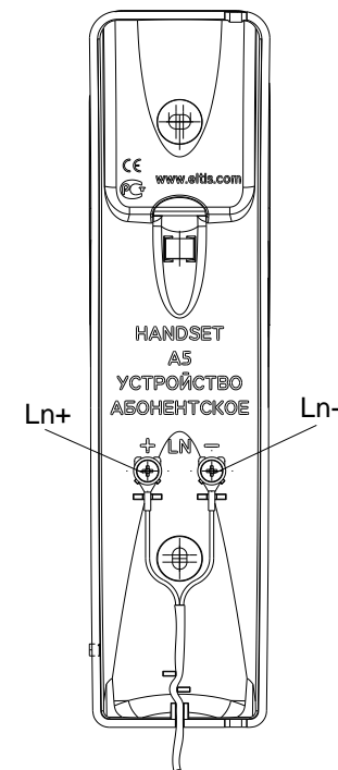
Рис.2 Клеммы подключения устройства абонентского А5.
